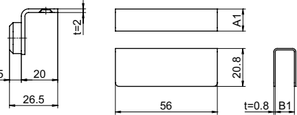
OT-B090-SUS用受金具
