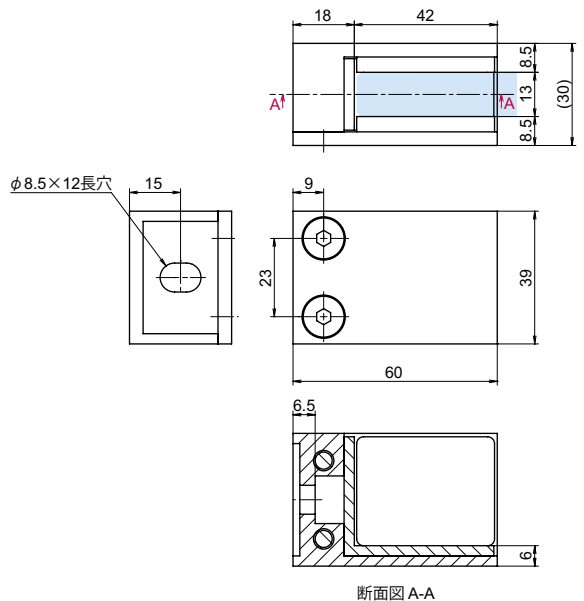
断面図 A-A
