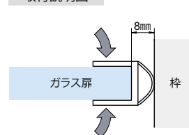
取付説明図
