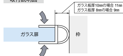
取付説明図
