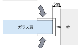
取付説明図
