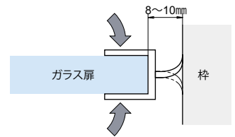
取付説明図
