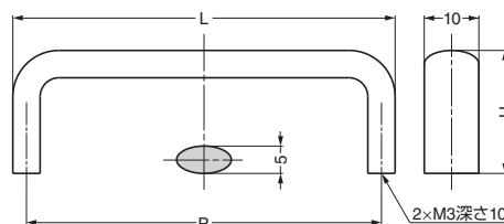
DS-50型、DS-70型、DS-90型
