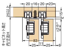
上レール 12 13 使用時 扉厚25mmの場合
