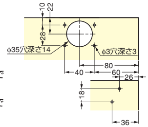
■扉の加工寸法
