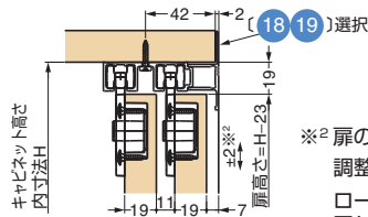
上レール 14 15 使用時 扉厚19mmの場合
