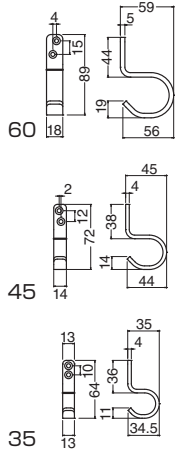
ST-210 ステンビームフック NEW (ステンレス/A4×25)
