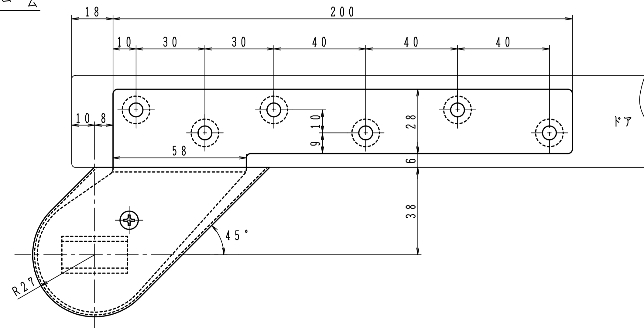
③ アーム
