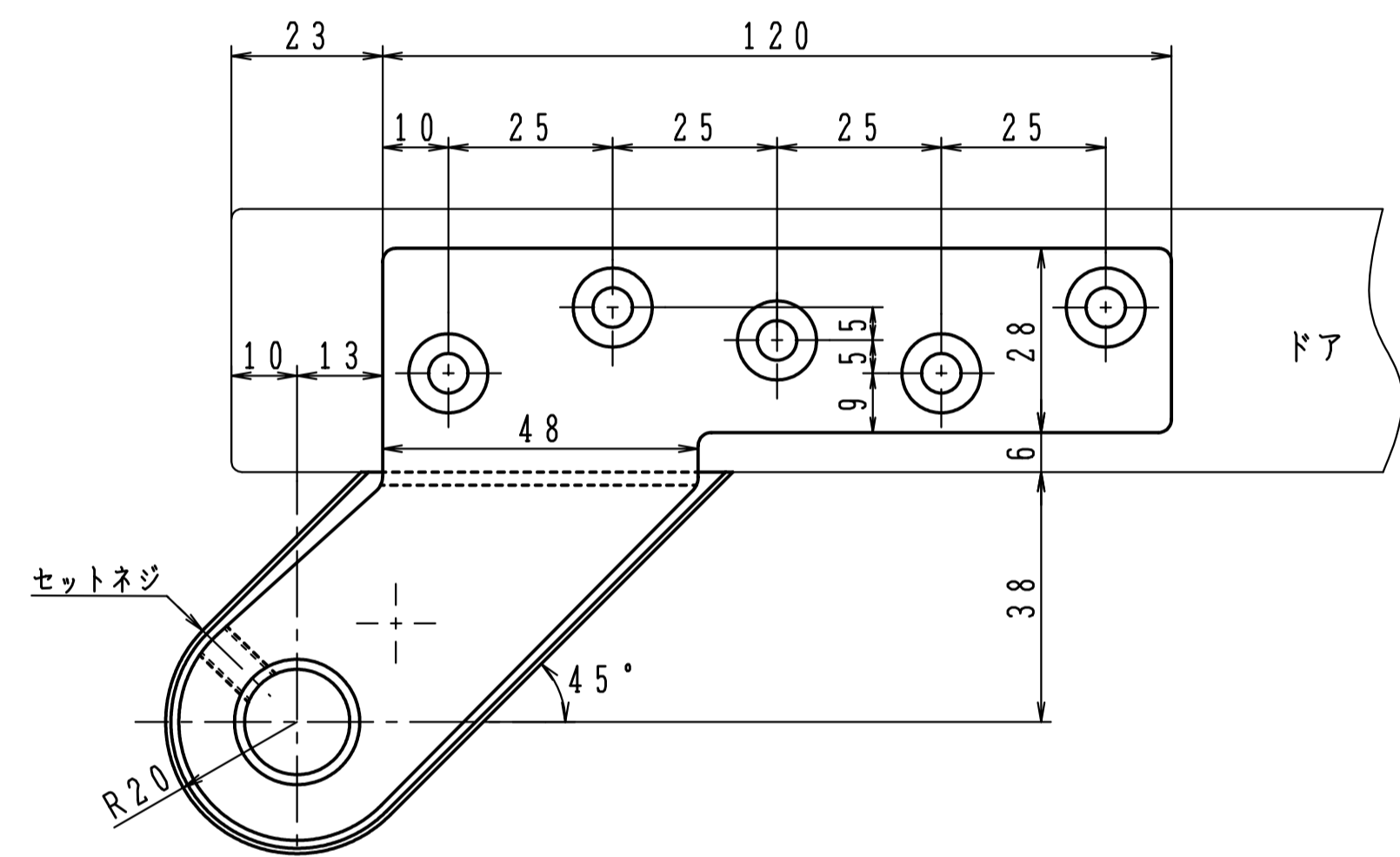
③ アーム
