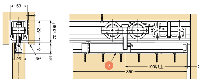
下ガイドレール⑩ 使用例
