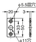
ストライクプレート
