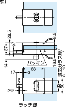
ラッチ錠
