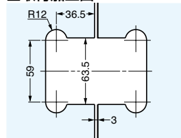
■取付加工図
