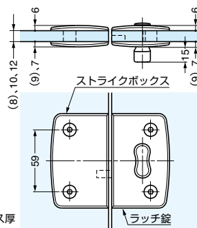
■取付加工図
