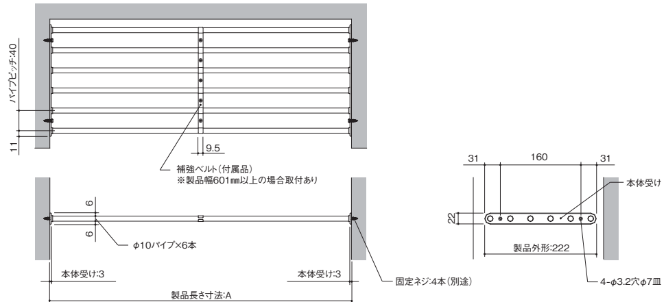
P96-6(パイプ6本) <横付けタイプ>
