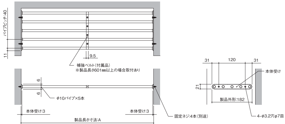
P95-5(パイプ5本) <横付けタイプ>
