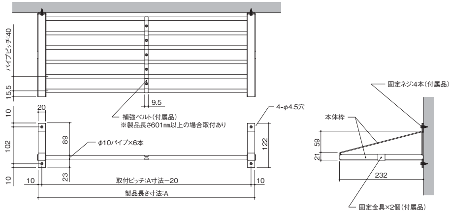
P94-6(パイプ6本) <バック付けタイプ>
