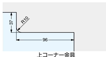
上コーナー金具
