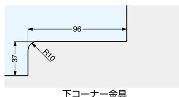
下コーナー金具
