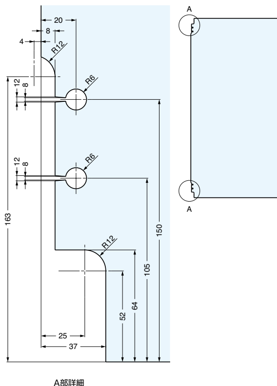
ガラス扉加工図
