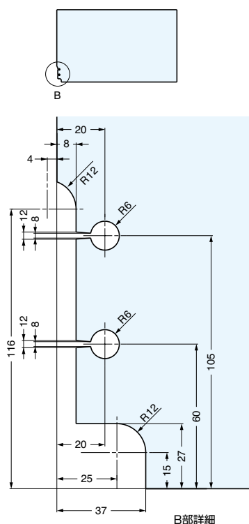
欄間加工図
