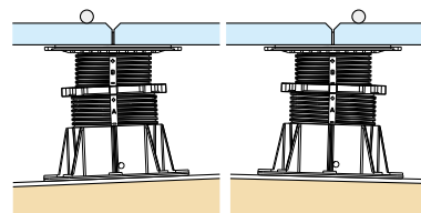
勾配調整機構付です (0～5%)
