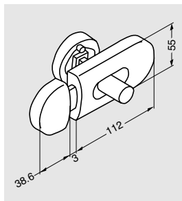
850-300の表示器
