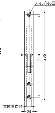
フロントパネル
