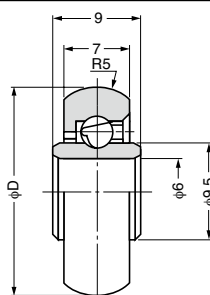
■内軸穴仕様
