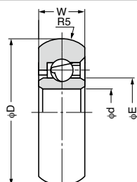
■内軸穴仕様
