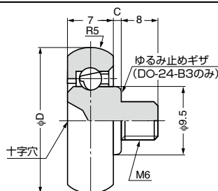
■ねじ軸仕様
