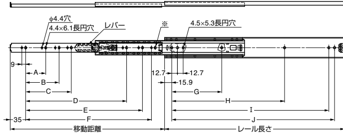
図中※印付の穴（インナーレールの一末端の長穴）は、取付穴として使用しないでください。
