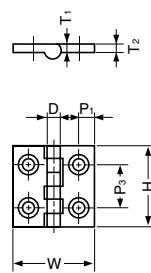
穴数=4の場合
