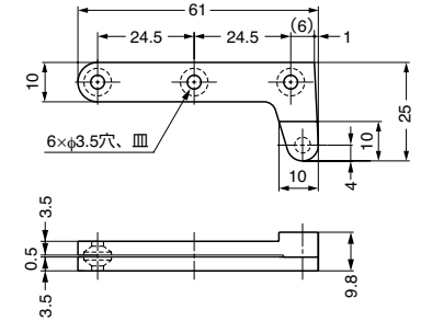
本図は右用を示します。
