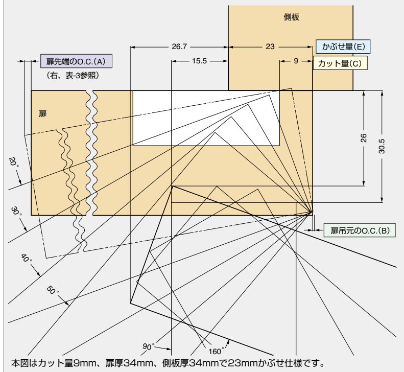
本図は、カット量9mm、扉厚34mm、23mmかぶせ仕様でH160-34/23、またはH160-C34/23(キャッチ付)とマウンティングプレート 100-03A(別売)の組み合わせです。
