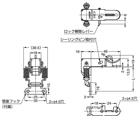
STF-C64A ばね付 ご使用時にパッキンは不要です。
