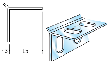
04018 かど定木D-3 1.82m/半透明/200本入
