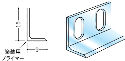
04005 したば定木9 プライマー付 1.82m/半透明/250本入
