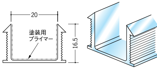
02009 溝メジ20 プライマー付 2m/半透明/100本入
