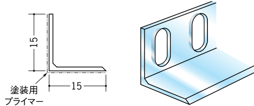
04007 したば定木15 プライマー付 1.82m/半透明/200本入
