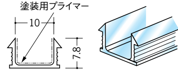
02007 溝メジ10 プライマー付 2m/半透明/200本入
