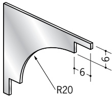
79053 アルミCRS-1 サイドキャップ アルマイトシルバー/t=1.0mm
