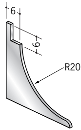
79054 アルミCRS-2 サイドキャップ アルマイトシルバー/t=1.0mm
