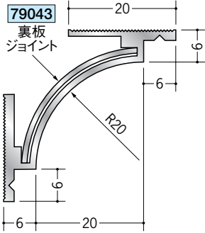
55049 アルミCRS-1 (廻り縁・入隅) 3m/アルマイトシルバー
