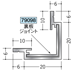
55171 アルミAD-1 (出隅) 3m/アルマイトシルバー
