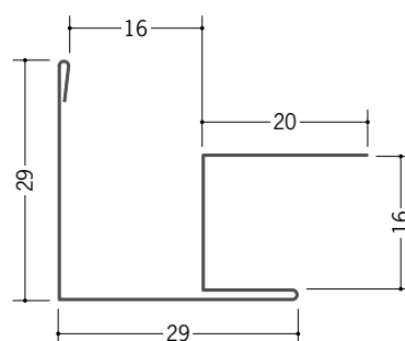
63155 亜鉛出隅15A 1.82m/アエンメッキ銅板/t=0.27
