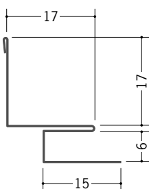
63156 亜鉛入隅5B 1.82m/アエンメッキ銅板/t=0.27
