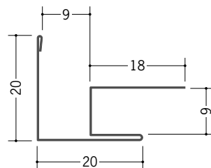
63152 亜鉛出隅8A 1.82m/アエンメッキ銅板/t=0.27
