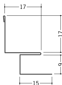
63158 亜鉛入隅8B 1.82m/アエンメッキ銅板/t=0.27
