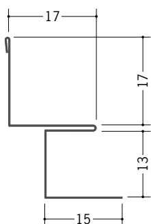
63160 亜鉛入隅12B 1.82m/アエンメッキ銅板/t=0.27
