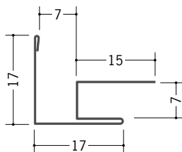
63151 亜鉛出隅6A 1.82m/アエンメッキ銅板/t=0.27
