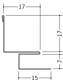
63157 亜鉛入隅6B 1.82m/アエンメッキ銅板/t=0.27
