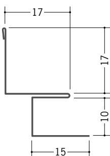
63159 亜鉛入隅9B 1.82m/アエンメッキ銅板/t=0.27
