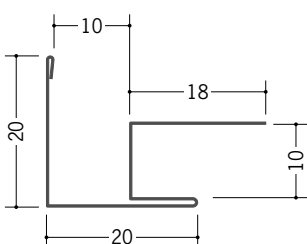
63153 亜鉛出隅9A 1.82m/アエンメッキ銅板/t=0.27
