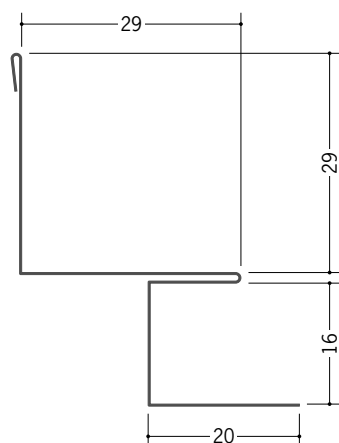
63161 亜鉛入隅15B 1.82m/アエンメッキ銅板/t=0.27
