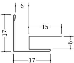
63150 亜鉛出隅5A 1.82m/アエンメッキ銅板/t=0.27
