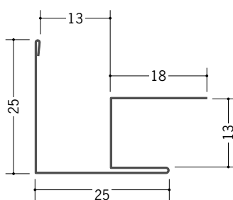
63154 亜鉛出隅12A 1.82m/アエンメッキ銅板/t=0.27
