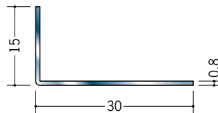
63138 ステンアンクル 0.8×15×30 2m/ヘアライン
