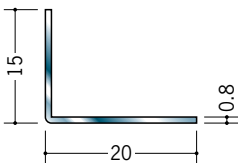
63136 ステンアンクル 0.8×15×20 2m/ヘアライン
