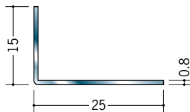
63137 ステンアンクル 0.8×15×25 2m/ヘアライン
