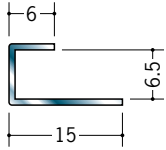
63103 ステンSCS-6.5 2m/ヘアライン/t=0.8
