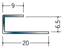
63120 ステンSCM-6 2m/ヘアライン/t=0.8
