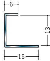
63106 ステンSCS-13 2m/ヘアライン/t=0.8
