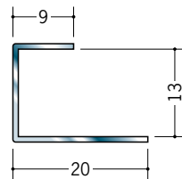
63123 ステンSCM-12 2m/ヘアライン/t=0.8
