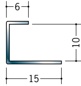
63105 ステンSCS-10 2m/ヘアライン/t=0.8
