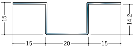
20088 ステンハット型HK-20 2.73m/ヘアライン/t=0.8
