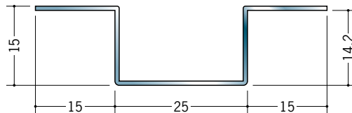
20089 ステンハット型HK-25 2.73m/ヘアライン/t=0.8
