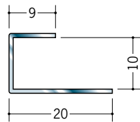
63122 ステンSCM-9 2m/ヘアライン/t=0.8
