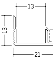
50137 アルミ12ABカラー 2.73m / バニラホワイト カスタムブラック
