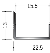
50138 アルミ15ABカラー 2.73m / バニラホワイト カスタムブラック
