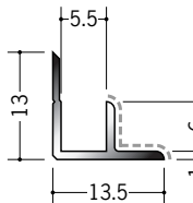
50132 アルミ5ABカラー 2.73m / バニラホワイト カスタムブラック
