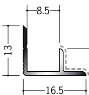
50134 アルミ8ABカラー 2.73m / バニラホワイト カスタムブラック
