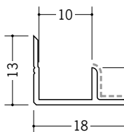
50135 アルミ9ABカラー 2.73m / バニラホワイト カスタムブラック
