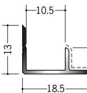
50136 アルミ10ABカラー 2.73m / バニラホワイト カスタムブラック
