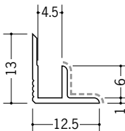
50131 アルミ4ABカラー 2.73m / バニラホワイト カスタムブラック
