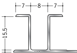
53072 アルミハット型15.5 2.5m/アルマイトシルバー
