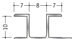
53074 アルミハット型9.5 2.5m/アルマイトシルバー
