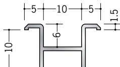
53186 アルミハット90MC 2.73m/アルマイトシルバー
