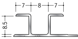
53070 アルミハット型8.5 2.5m/アルマイトシルバー
