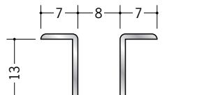
53071 アルミハット型13 2.5m/アルマイトシルバー
