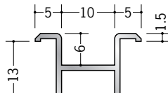
53187 アルミハット120MC 2.73m/アルマイトシルバー
