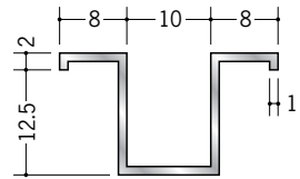
53089 アルミハット12.5×10 3m/アルマイトシルバー
