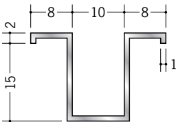
53090 アルミハット15×10 3m/アルマイトシルバー
