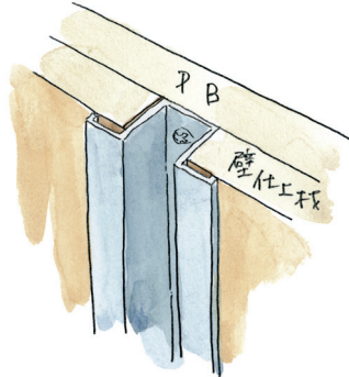
53060 アルミHJ-1215 3m/アルマイトシルバー
