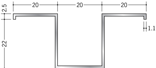
53202 アルミハット22 2.5m/アルマイトシルバー
