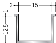
53060 アルミHJ-1215 3m/アルマイトシルバー
