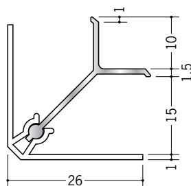
58060 アルミAKI-15.5 2.73m/アルマイトシルバー ベース:ビニール
