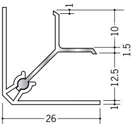
58080 アルミAKI-12.5 2.73m/アルマイトシルバー ベース:ビニール
