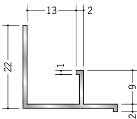
54172 アルミF型入隅13 3m/アルマイトシルバー
