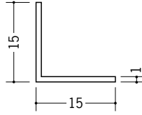
36010 アングル15 (t=1.0) 1.82m/ホワイト/200本入 2.73m/ホワイト/150本入
