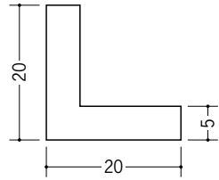
36191 アングル20 (t=5.0) 2.73m/ホワイト/20本入
