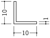
36004 アングル10 1.82m/ホワイト/300本入 2.73m/ホワイト/250本入
