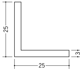
36182 アングル25 (t=3.0) 1.82m/ホワイト/40本入 2.73m/ホワイト/25本入
