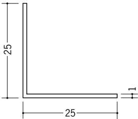
36109 アングル25 (t=1.0) 1.82m/ホワイト/150本入 2.73m/ホワイト/100本入
