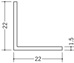
36008 アングル22 (t=1.5) 1.82m/ホワイト/100本入 2.73m/ホワイト/70本入
