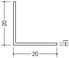
36107 アングル20 (t=1.0) 1.82m/ホワイト/150本入 2.73m/ホワイト/100本入
