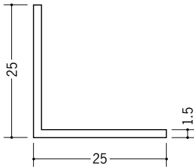
36009 アングル25 (t=1.5) 1.82m/ホワイト/100本入 2.73m/ホワイト/70本入
