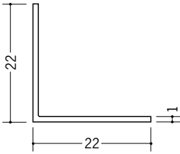
36108 アングル22 (t=1.0) 1.82m/ホワイト/150本入 2.73m/ホワイト/100本入
