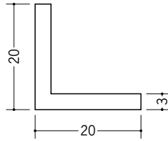
36181 アングル20 (t=3.0) 1.82m/ホワイト/50本入 2.73m/ホワイト/40本入
