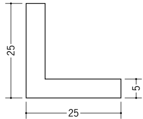
36192 アングル25 (t=5.0) 2.73m/ホワイト/15本入
