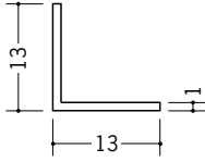
36005 アングル13 1.82m/ホワイト/300本入 2.73m/ホワイト/200本入
