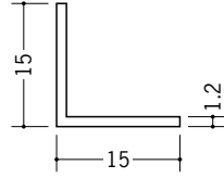
36006 アングル15 (t=1.2) 1.82m/ホワイト/200本入
