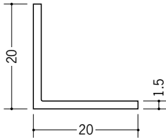
36007 アングル20 (t=1.5) 1.82m/ホワイト/100本入 2.73m/ホワイト/70本入
