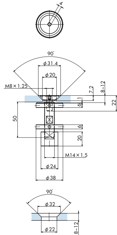
ガラスカット寸法 Cut out dimensions
