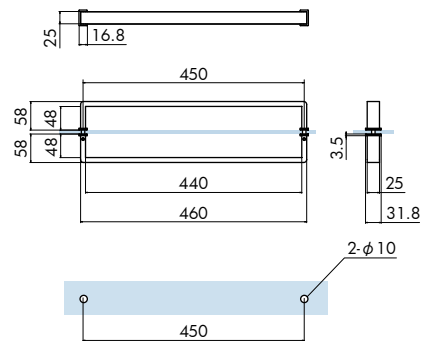
ガラスカット寸法 Cut out dimensions
