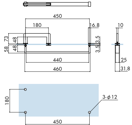
ガラスカット寸法 Cut out dimensions
